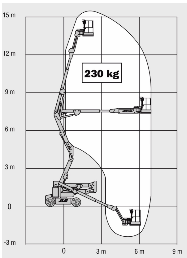
JLG E450AJ
